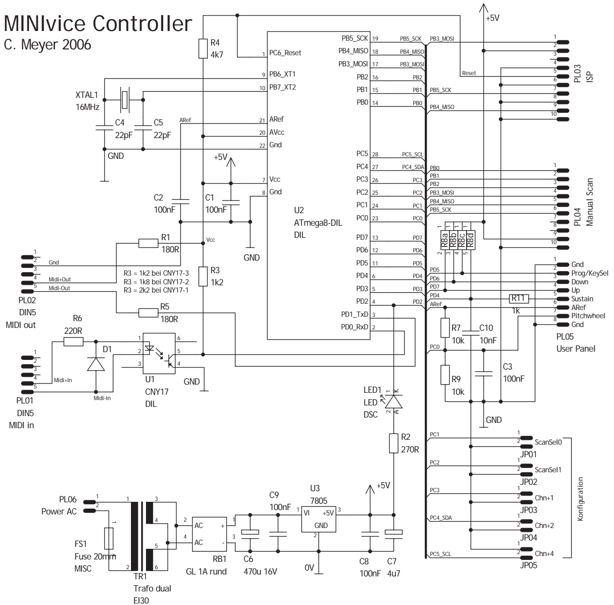
Schaltplan MINIvice Controller-Platine
