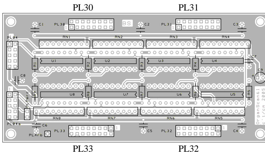
Bestückungs- und Anschlussplan Scan-Platine OrganScan61
